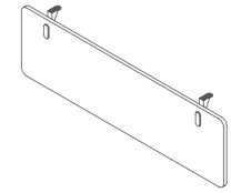
Hanging Modesty Panel M10B-HMP-0935 900×T18×H350(fit W1400 Desk) M10B-HMP-1135 1100×T18×H350(fit W1600 Desk) M10B-HMP-1335 1300×T18×H350(fit W1800 Desk) M10B-HMP-1635 1600×T18×H350(fit W2100 Desk)
