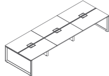
Six Persons Workstation-type B M10-MB6-1206 3600×1200×H750 M10-MB6-1407 4200×1400×H750 M10-MB6-1507 4500×1400×H750 M10-MB6-1608 4800×1600×H750
