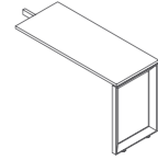
Return M10-DR2-0905 900×500×H750 M10-DR2-1205 1200×500×H750
