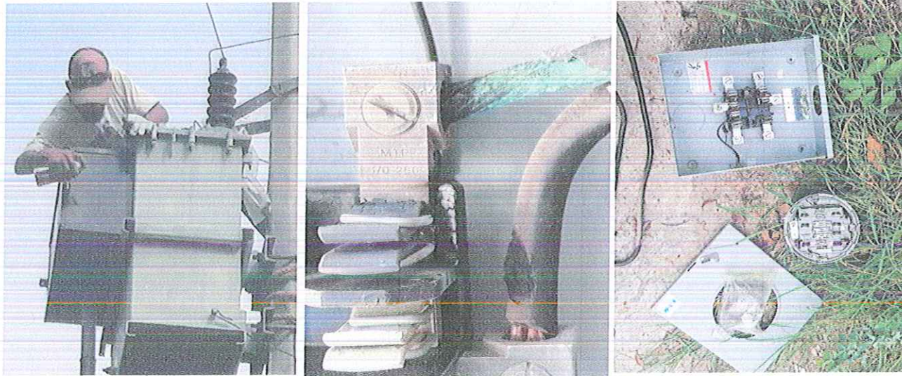
LIBRANZA ALTA TENSION , LIMPIEZA CON SOLVENTE DIELECTRICO,REAPRIETE DE TORNILLERIA,BOQUILLAS ALTA Y BAJA TENSION A SUBESTACION TIPO POSTE 45 KVA ,SUMINISTRO DE BASE 7X200,CABLE 1/0 ,SUMINISTRO DE SISTEMA DE TIERRAS, TUBERIA CONDUIT Y CABLEADO 12 AWG, MANTENIMIENTO A ARRANCADOR A TENSION REDUCIDA 30 HP/220V,PRUEBAS DE PUESTA EN SERVICIO DE UNA BOMBA SUMERGIBLE 30HP/220V
