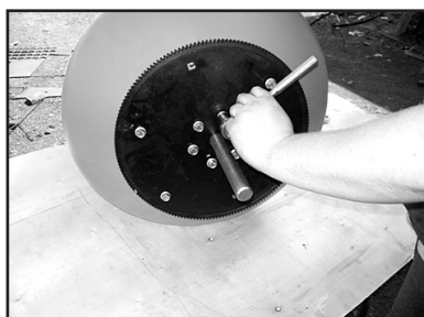
Step 13 • Paso 13 • Étape 13 Install bolts leaving out the three that do not have nuts welded to the inside • Instale los tornillos, dejando fuera los tres que no tienen tuercas soldadas en el interior • Installez les boulons en laissant les trois qui n'ont pas d'écrous soudés à l'intérieur
