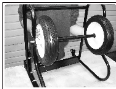
Step 3 • Paso 3 • Étape 3 Install Wheels as shown, pushing axle rod end out and the other end into the frame • Instale las ruedas como se muestra, empujando hacia afuera el extremo de la varilla del eje y el otro extremo dentro del chasis • Installez les roues conformément à l'illustration, en poussant l'extrémité de la tige de l'essieu vers l'extérieur et l'autre extrémité dans le châssis
