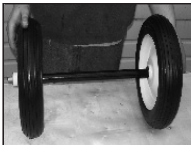
Step 2 • Paso 2 • Étape 2 With the long end of wheel hub facing out assemble. • Con el extremo largo del cubo de la rueda viendo hacia el conjunto • Avec l'extrémité longue du moyeu de la roue dirigée dans l'autre sens du montage
