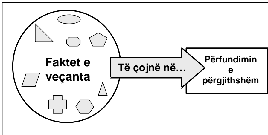
Figura 1.2 Metoda induktive
