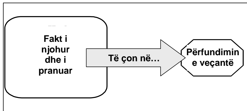
Figura 1.1 Arsyetimi deduktiv
