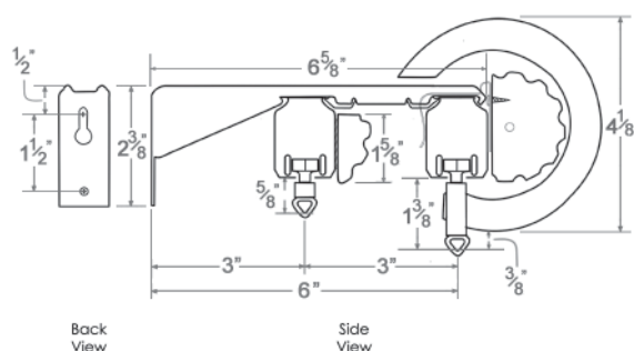
EZ51 6" EasyPull™ Double Bracket
