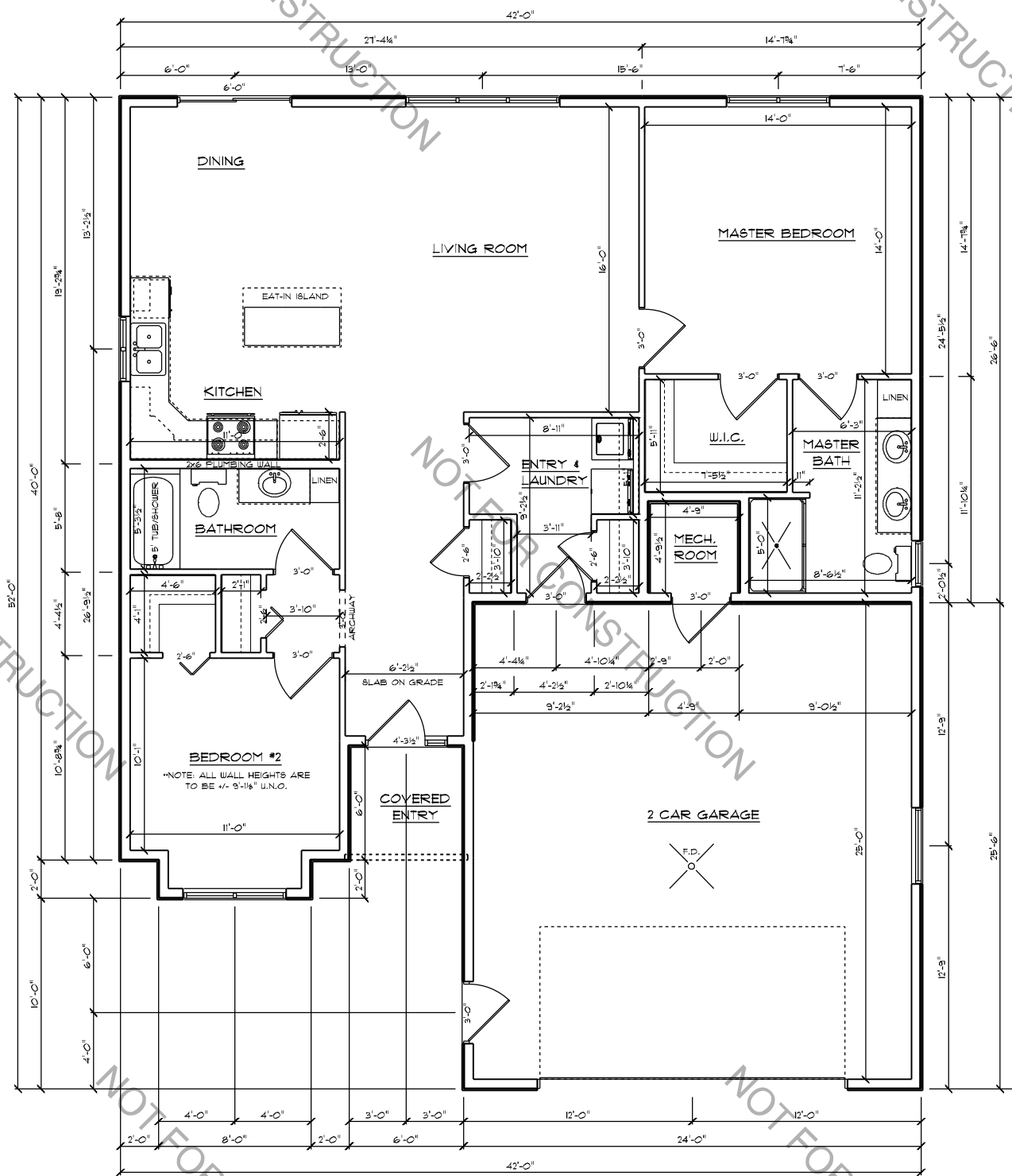
FLOOR PLAN SCALE: 1/8" = 1'-0"
