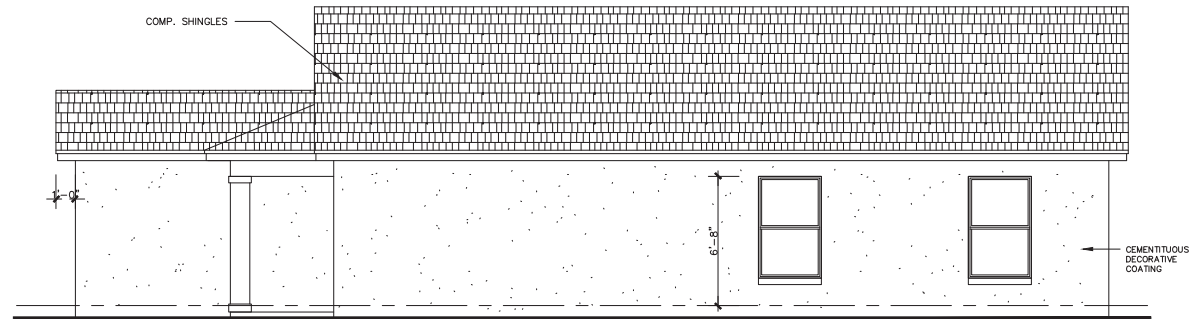
RIGHT ELEVATION
