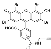
(D) Eosin alkyne
