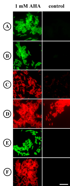
(D) Eosin alkyne
