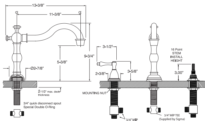
Roman Tub Set (Quick Connect)
