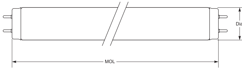
T8 & T10 Med Bi-Pin G13 Base
