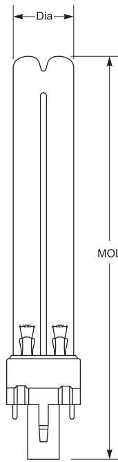
G23 Base
