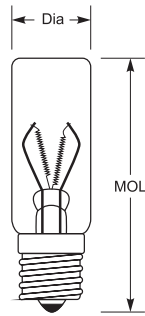
E17 Base
