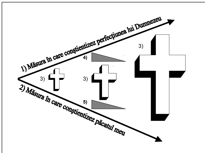
Figura 5.1 Diagrama Crucii
