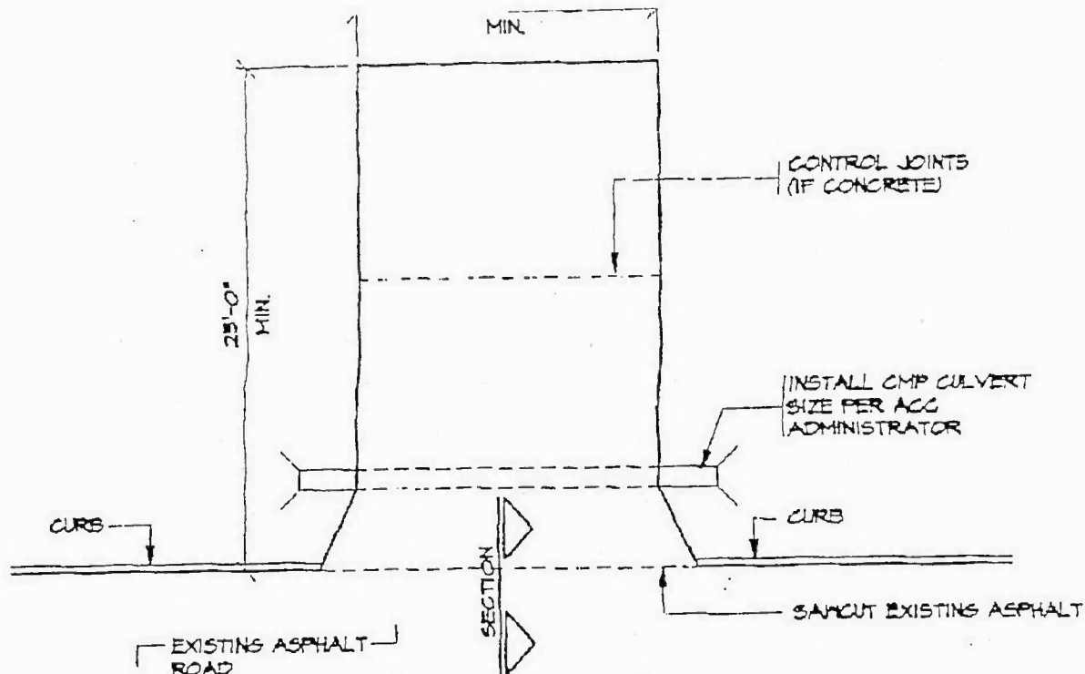
PLAN VIEW SCALE: 1/8" = 1'-0"
