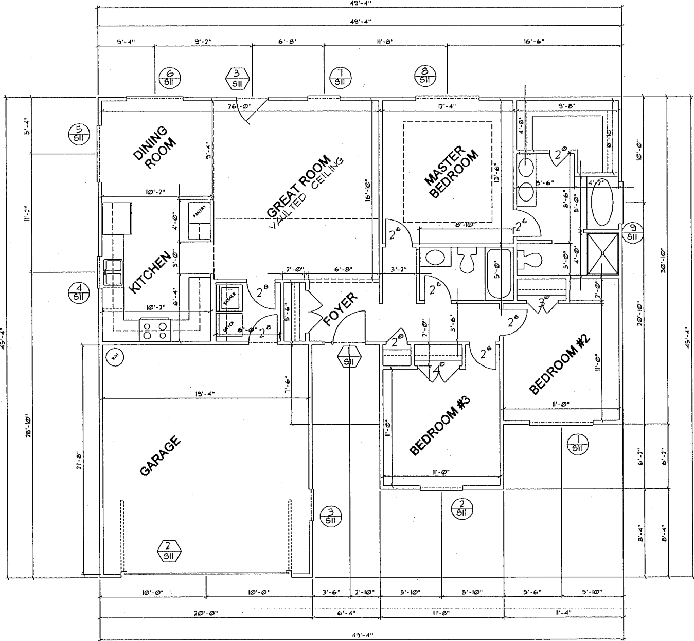
FLOOR PLAN 11 X 17 FORMAT SCALE: 1/8" = 1'-0" 24 X 36 FORMAT SCALE: 1/4" = 1'-0"
