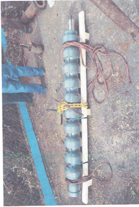
1.- SUMINISTRO DE UN CUERPO DE BOMBA VERTICAL TIPO TURBINA, 75 HP., MODELO 10ALS1.9 DESCARGA EN 6" DIA, MARCA AS PUMIS
