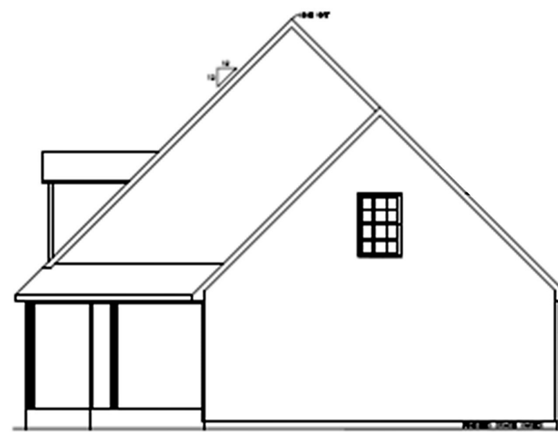
RIGHT ELEVATION
