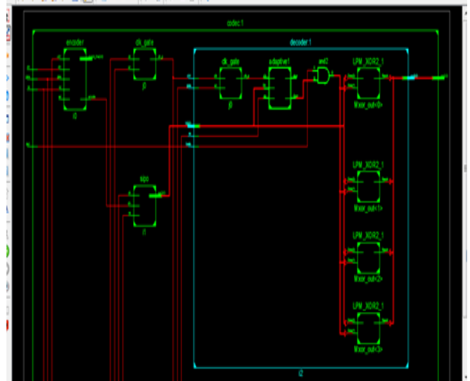
Fig. 6. RTL Schematic
