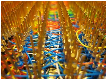
WIRE WRAPPING
