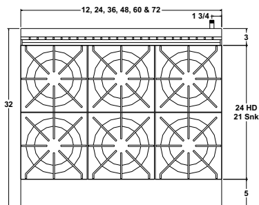
Model: IDR-4G24
