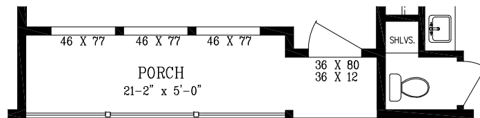
OPTIONAL ENTRY
