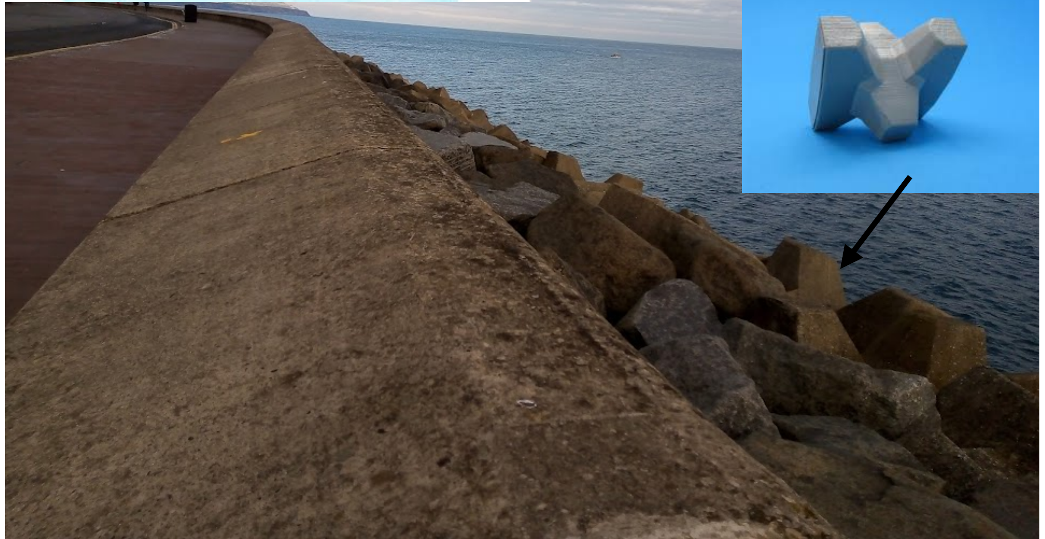
ACCROPODE
