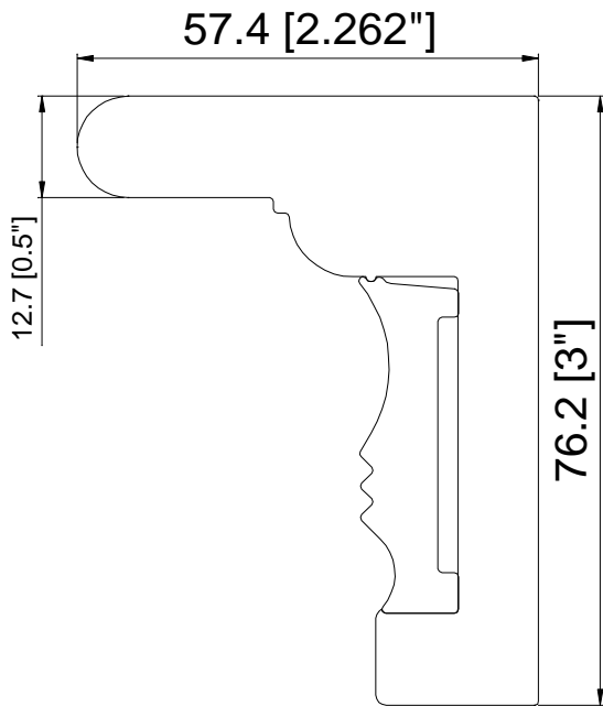
3" Deco Sill Frame
