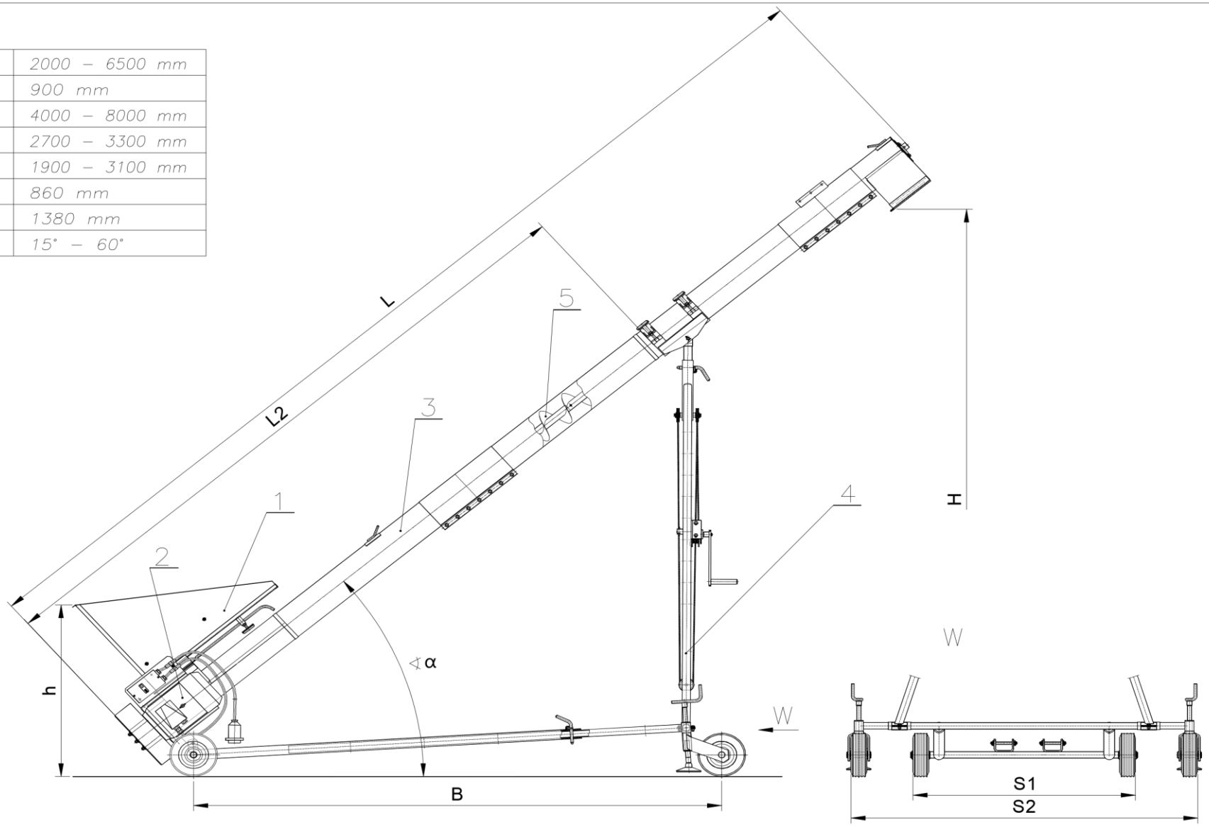
Figura. 1 Tornillo T 206/4
