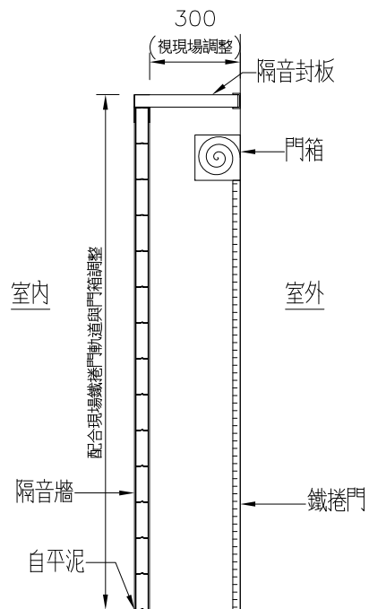
立剖圖
