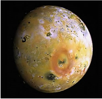
Jupiter's Moon Io
