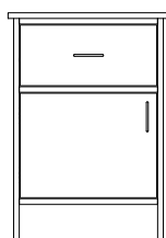
1 Drawer/1 Door Bedside 21" W, 18" D, 30" H (CEN-125)
