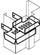
METAL OR WOOD STUD ANCHOR
