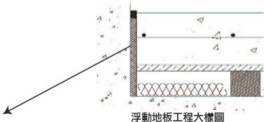
側邊防振板貼附於RC邊墩上
