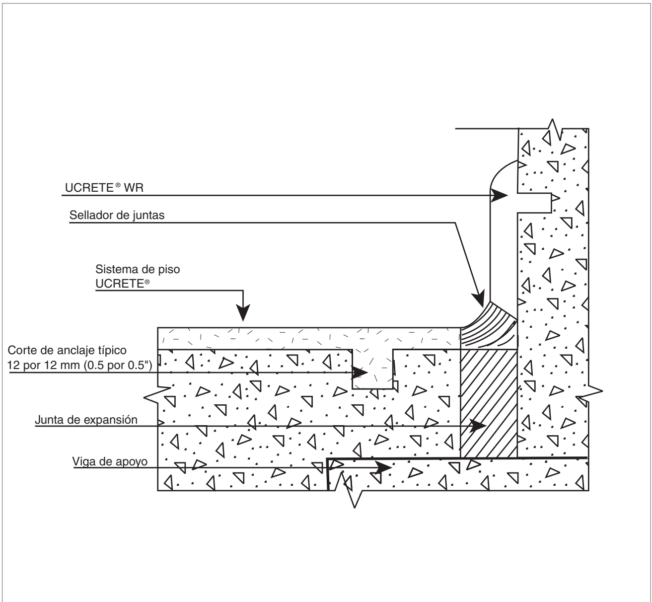
FIGURA 5 Sistema de Pisos UCRETE®
