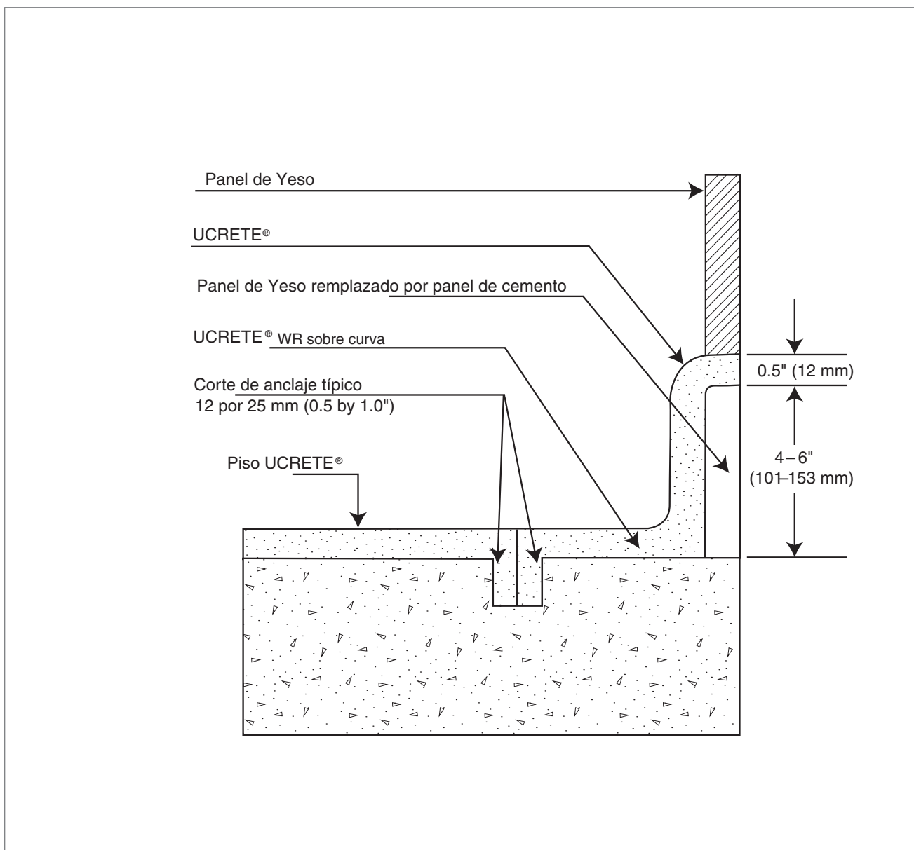
FIGURA 13 Sistema de Pisos UCRETE®
