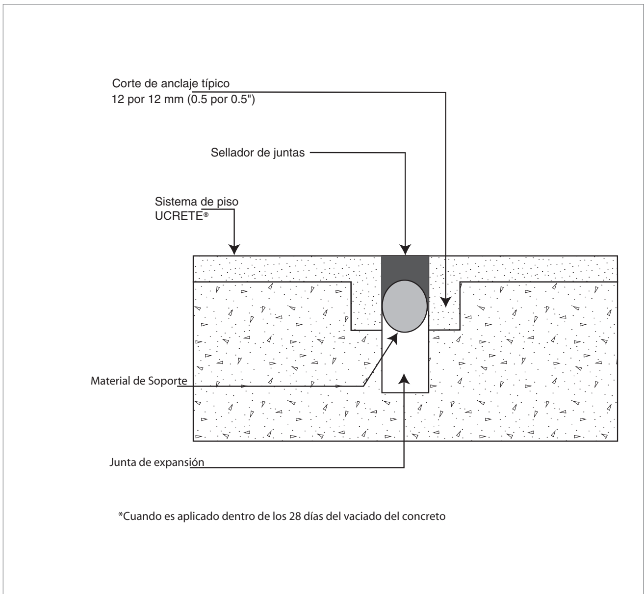
FIGURA 7 Sistema de Pisos UCRETE®
