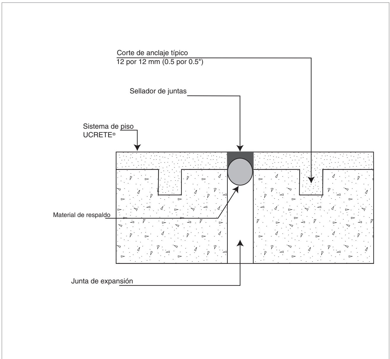
FIGURA 6 Sistema de Pisos UCRETE®
