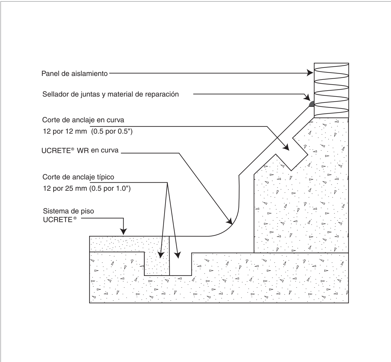
FIGURA 3 Sistema de Pisos UCRETE®
