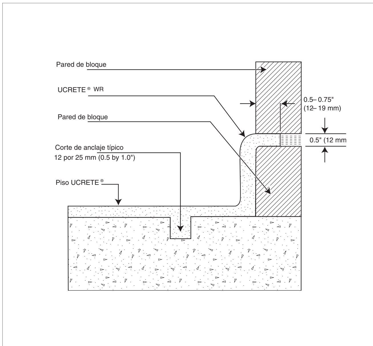
FIGURA 14 Sistema de Pisos UCRETE®
