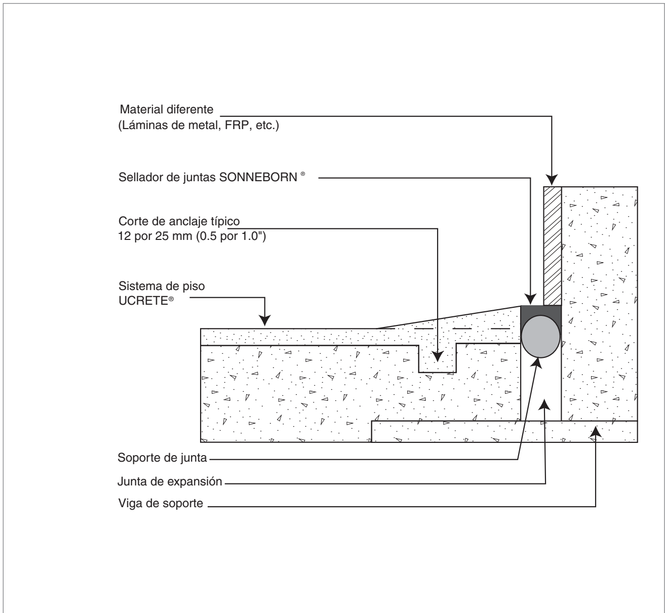
FIGURA 4A Sistema de Pisos UCRETE®
