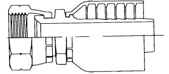
SAE 45° SWIVEL 10843
