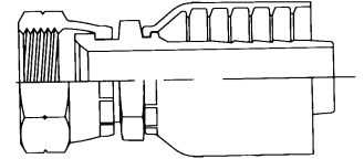
SAE 45° SWIVEL 10843
