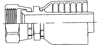
JIC 37° SWIVEL 10671
