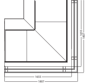
AVANTURIN MT 90° DIŞ KÖŞE / EXTERNAL CORNER
