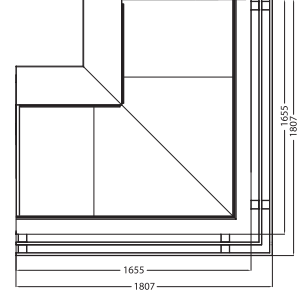
AVANTURIN DL 90° DIŞ KÖŞE / EXTERNAL CORNER
