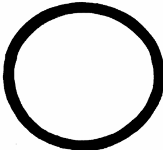
13452 QTY. 5 2-3/8 ID 2-3/4 OD
