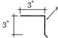
Eave Drip EF3
