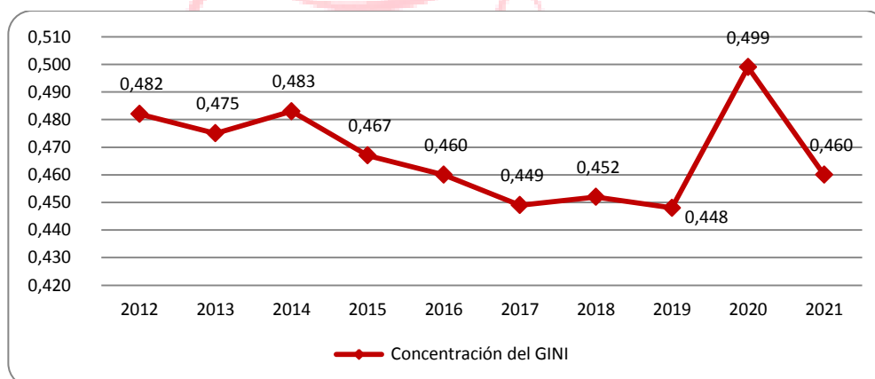
Concentración del GINI Período 2012 - 2021 Cartagena de Indias
