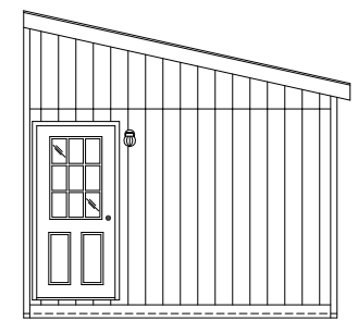
OPTIONAL FRONT ENDWALL DOOR
