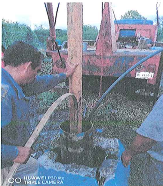
MONTAJE ELECTROMECANICO DE UNA BOMBA SUMERGIBLE 30 HP/220V- 84 MT DE COLUMNA ACERO AL CARBON 4",EN BOMBEO POZO PROFUNDO 1 MYO LOCALIZADO EN LA COL. 1 MYO DE ESTA CD. IGUALA GRO
