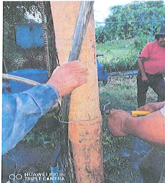
MONTAJE ELECTROMECANICO DE UNA BOMBA SUMERGIBLE 30 HP/220V- 84 MT DE COLUMNA ACERO AL CARBON 4", EN BOMBEO POZO PROFUNDO 1 MYO LOCALIZADO EN LA COL. 1 MYO DE ESTA CD. IGUALA GRO
