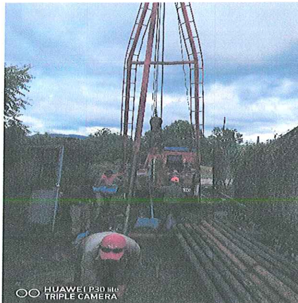
MONTAJE ELECTROMECANICO DE UNA BOMBA SUMERGIBLE 30 HP/220V- 84 MT DE COLUMNA ACERO AL CARBON 4", EN BOMBEO POZO PROFUNDO 1 MYO LOCALIZADO EN LA COL. 1 MYO DE ESTA CD. IGUALA GRO
