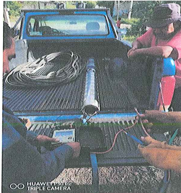
MONTAJE ELECTROMECANICO DE UNA BOMBA SUMERGIBLE 30 HP/220V- 84 MT DE COLUMNA ACERO AL CARBON 4", EN BOMBEO POZO PROFUNDO 1 MYO LOCALIZADO EN LA COL. 1 MYO DE ESTA CD. IGUALA GRO
