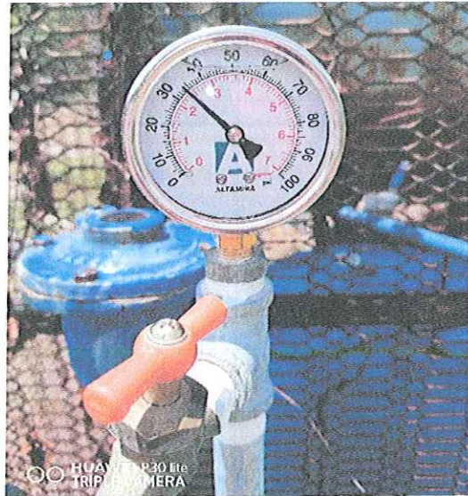
MONTAJE ELECTROMECHANICO DE UNA BOMBA SUMERGIBLE 30 HP/220V- 84 MT DE COLUMNA ACERO AL CARBON 4", EN BOMBEO POZO PROFUNDO 1 MYO LOCALIZADO EN LA COL. 1 MYO DE ESTA CD. IGUALA GRO.
