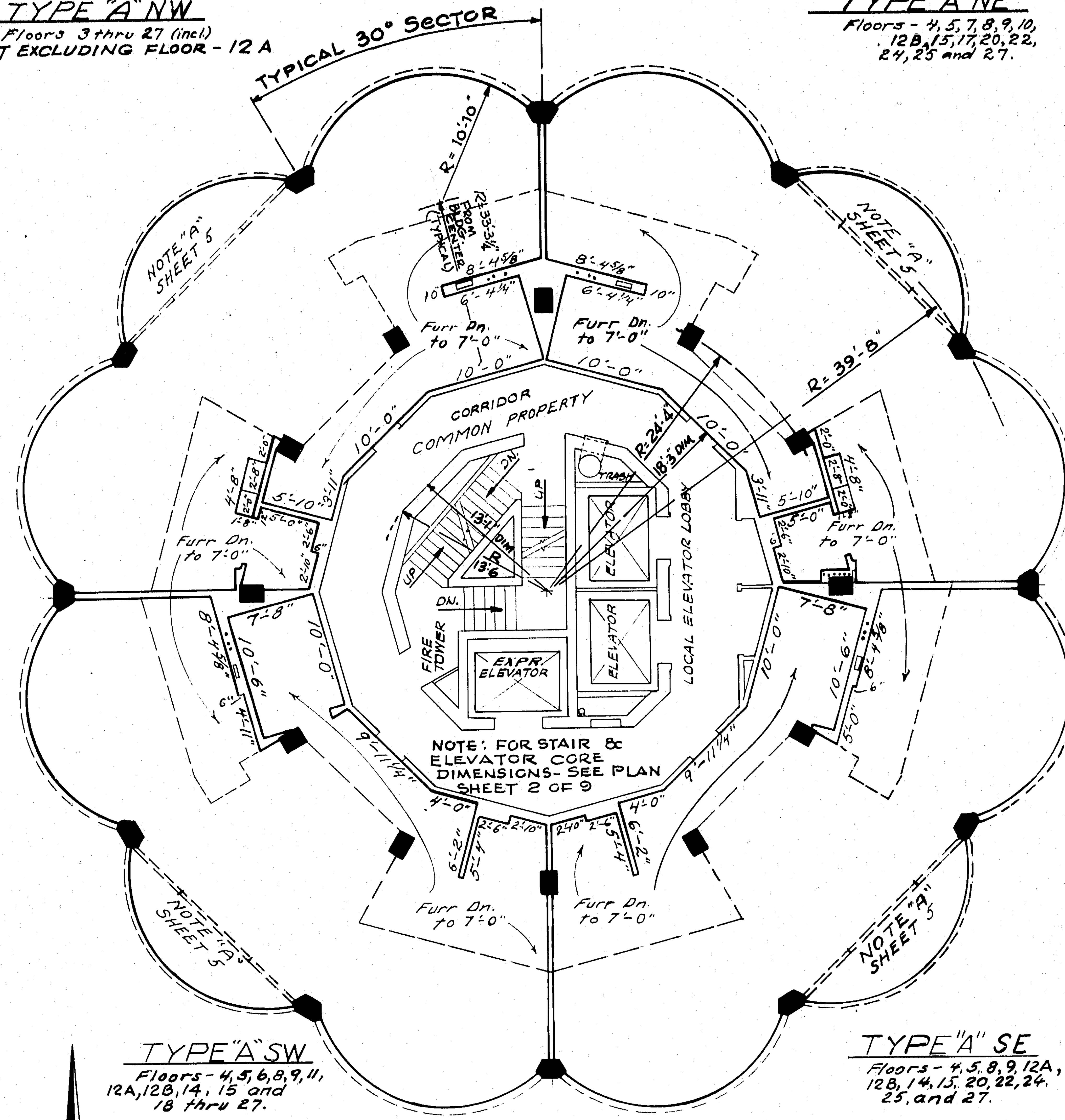
4- TYPE "A" Scale: 1/8" = 1'-0"
