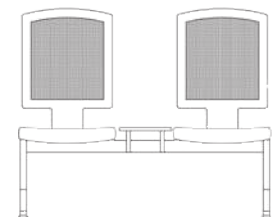
- REKS 322 F Genişlik-Width:100 cm Derinlik-Depth:68 cm Yükseklik-Height:91cm
