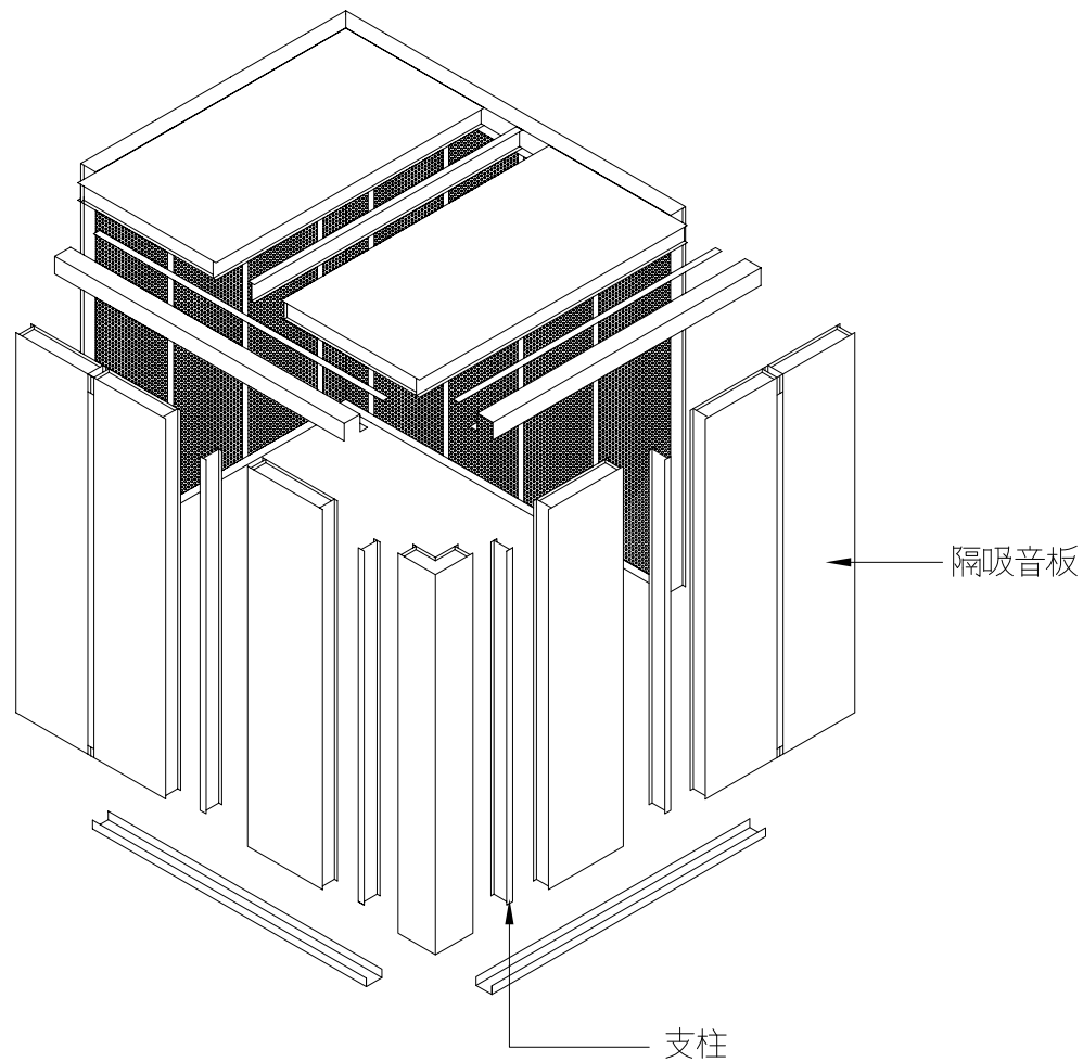
隔吸音板APC100(含烤漆)
