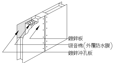
隔吸音板APC100(含烤漆)
