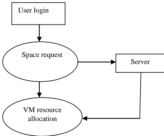
Fig. 2. SLA prediction
