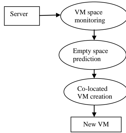
Fig. 4. VM migration
