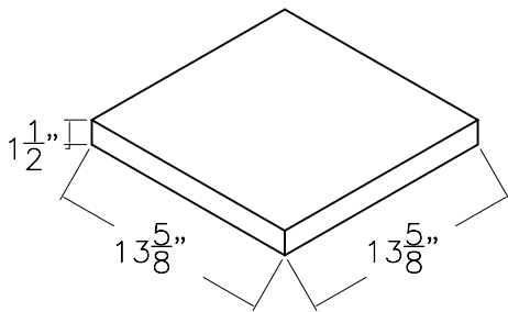
DT-1414 PAVER
