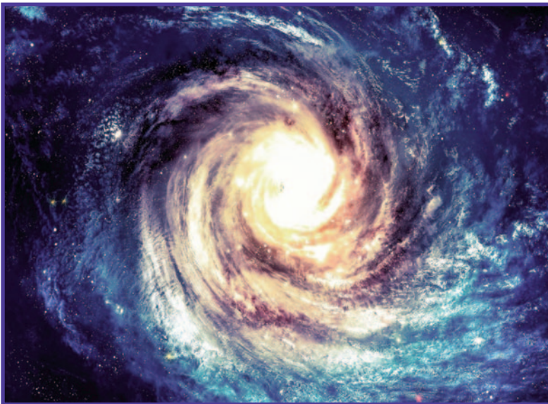
Andromeda Galaxy (NASA)
