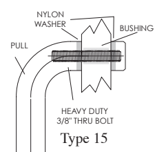
Type 15 Glass Door Thru Bolt
