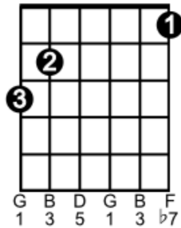
G 7
