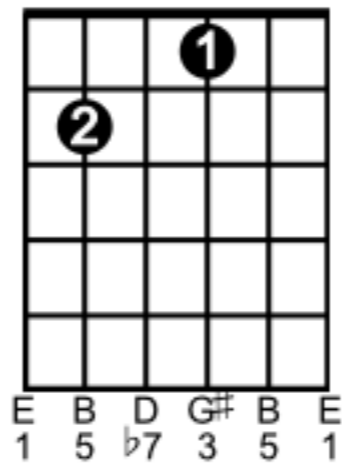
E 7
