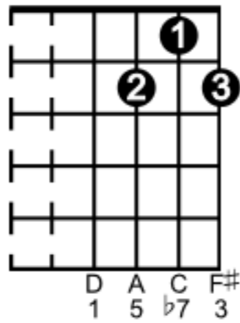
D 7
