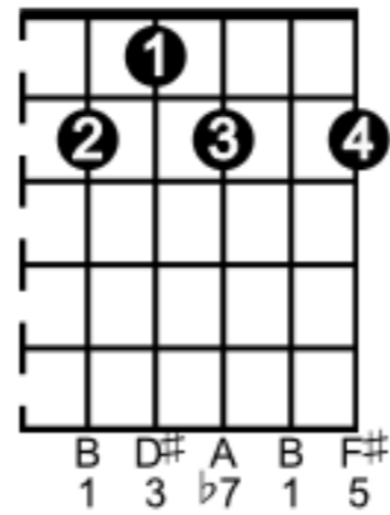
B 7
