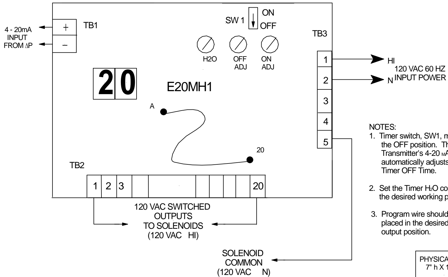
E20MH1, 20 POSITION TIMER 4 - 20 mA MODE
