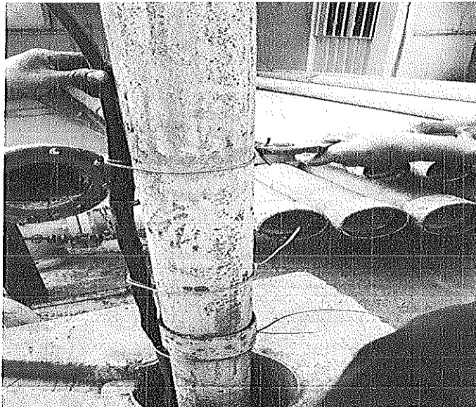
"SUMINISTRO, MONTAJE ELECTROMECANICO Y PRUEBAS DE UNA MOTOBOMBA SUMERGIBLE 40HP/440 V-150 MTS DE COLUMNA ACERO AL CARBON 6", EN BOMBEO POZO PROFUNDO 1, LOCALIZADO EN MAYA No. 1 OFICINAS DE CAPAMI, EN LA CIUDAD DE IGUALA GRO".
