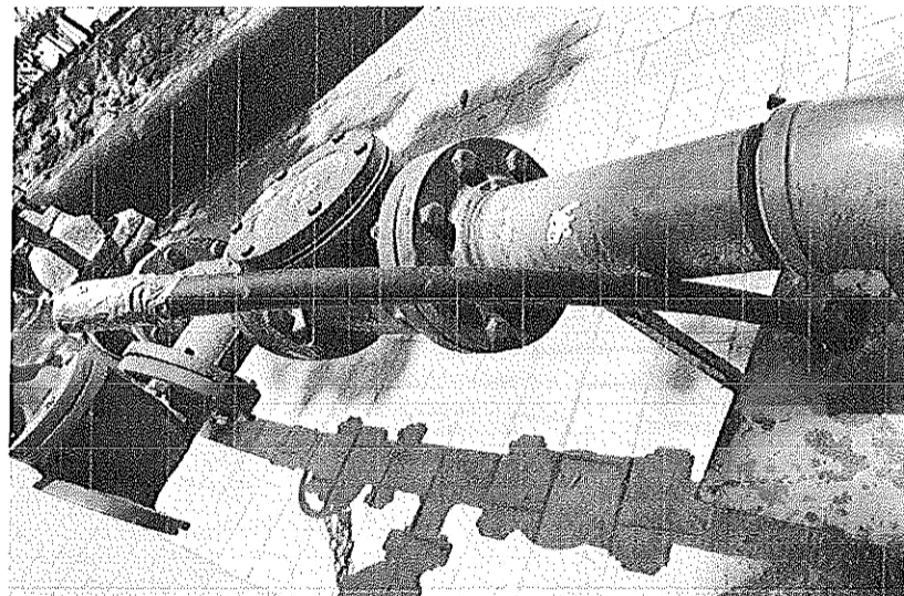
"SUMINISTRO, MONTAJE ELECTROMECANICO Y PRUEBAS DE UNA MOTOBOMBA SUMERGIBLE 40HP/440 V-150 MTS DE COLUMNA ACERO AL CARBON 6", EN BOMBEO POZO PROFUNDO 1, LOCALIZADO EN MAYA No. 1 OFICINAS DE CAPAMI, EN LA CIUDAD DE IGUALA GRO".
