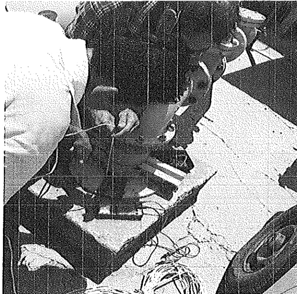
"SUMINISTRO, MONTAJE ELECTROMECANICO Y PRUEBAS DE UNA MOTOBOMBA SUMERGIBLE 40HP/440 V-150 MTS DE COLUMNA ACERO AL CARBON 6", EN BOMBEO POZO PROFUNDO 1, LOCALIZADO EN MAYA No. 1 OFICINAS DE CAPAMI, EN LA CIUDAD DE IGUALA GRO".
