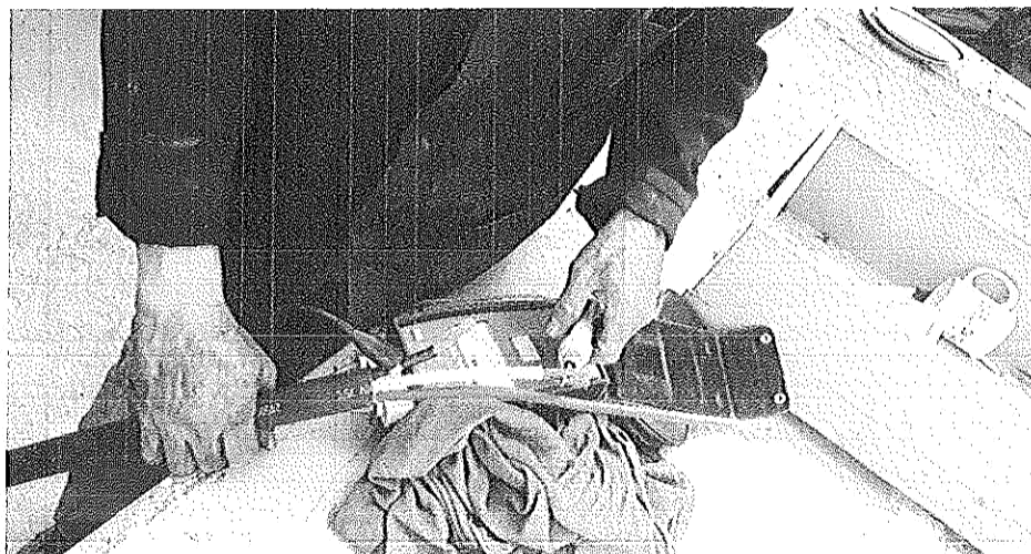
"SUMINISTRO, MONTAJE ELECTROMECANICO Y PRUEBAS DE UNA MOTOBOMBA SUMERGIBLE 40HP/440 V-150 MTS DE COLUMNA ACERO AL CARBON 6 ", EN BOMBEO POZO PROFUNDO 1, LOCALIZADO EN MAYA No. 1 OFICINAS DE CAPAMI, EN LA CIUDAD DE IGUALA GRO".
