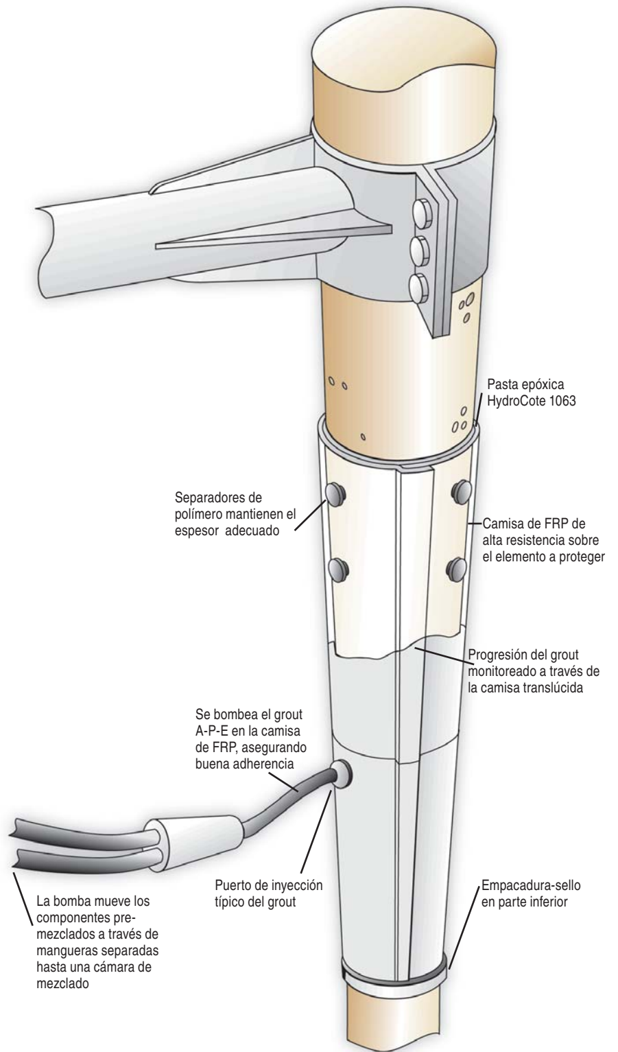
Camisa A-P-E para pilotes H
