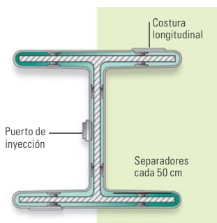
Camisa A-P-E para pilotes H
