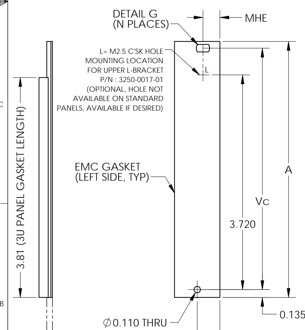
3U X 4HP
