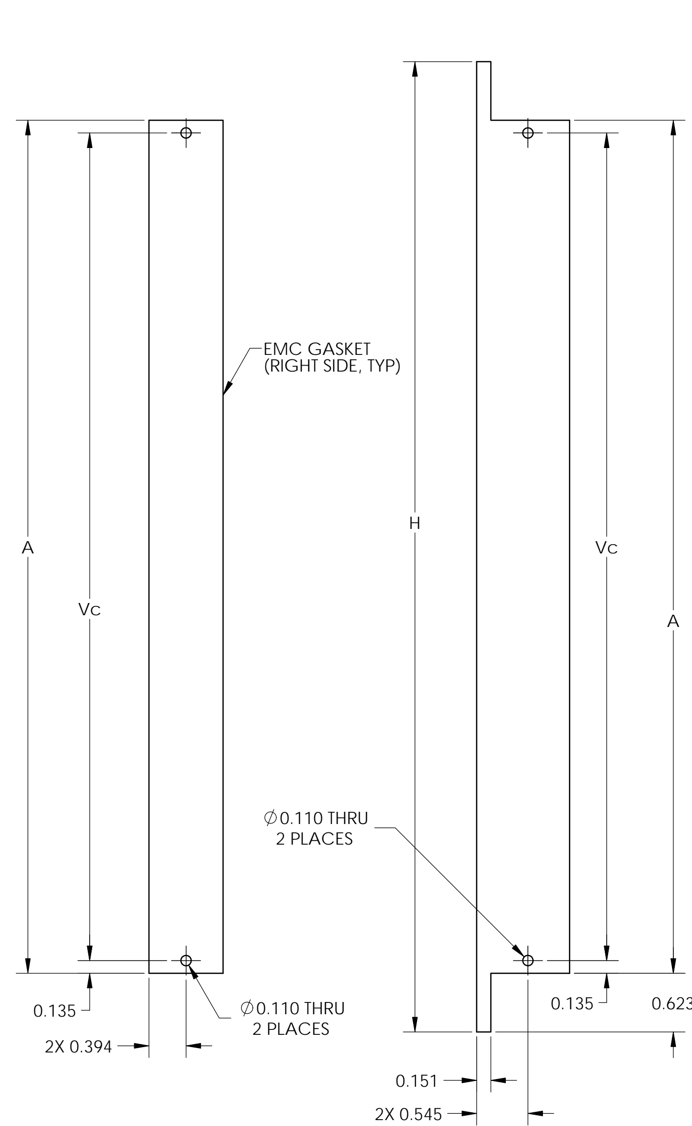
6U or 9U X 4HP
