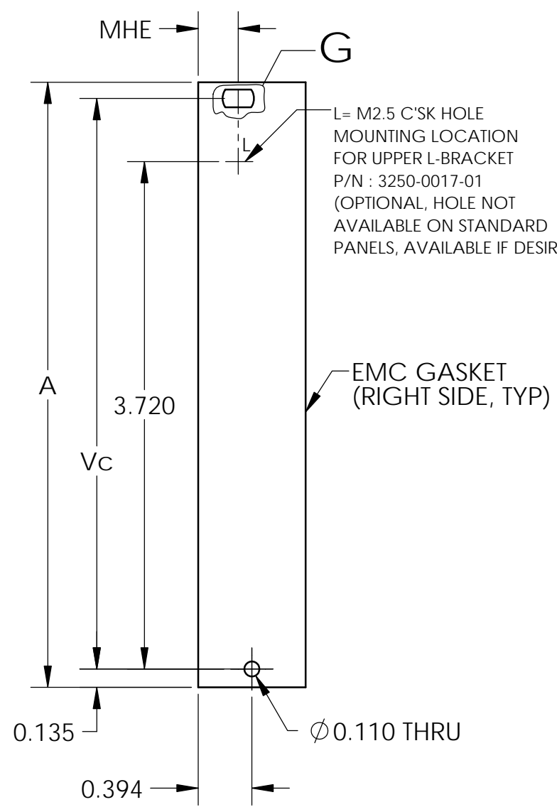
3U X 4HP
