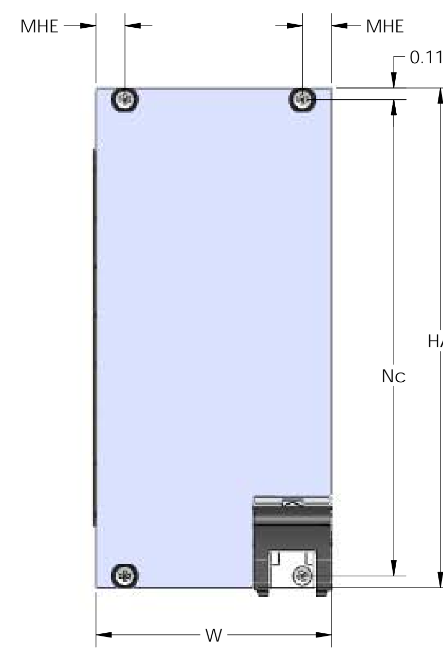
3U X 12HP
