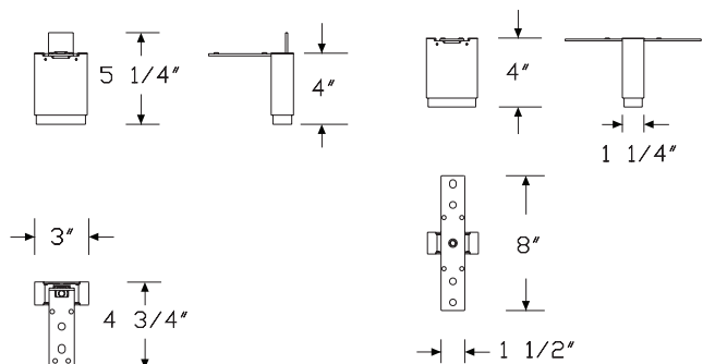
End of frame (1A)
