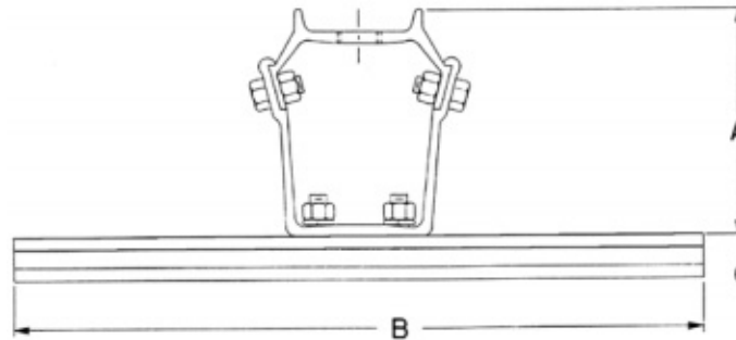
4 WAY T-SLOT
